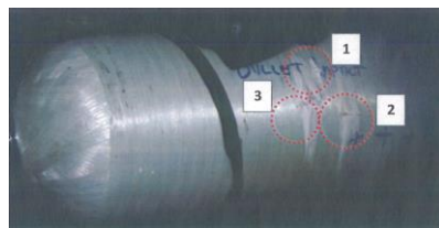
Prueba Balística con Proyectoil Calibre 50 AP Incendiario
