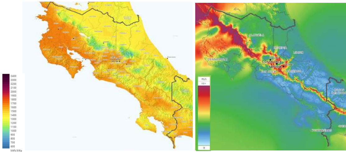
Figura 8. Mapa del potencial solar (izquierda) y eólico (derecha) de Costa Rica. Fuente: World Bank (2022), Global Solar Atlas y Global Wind Atlas
