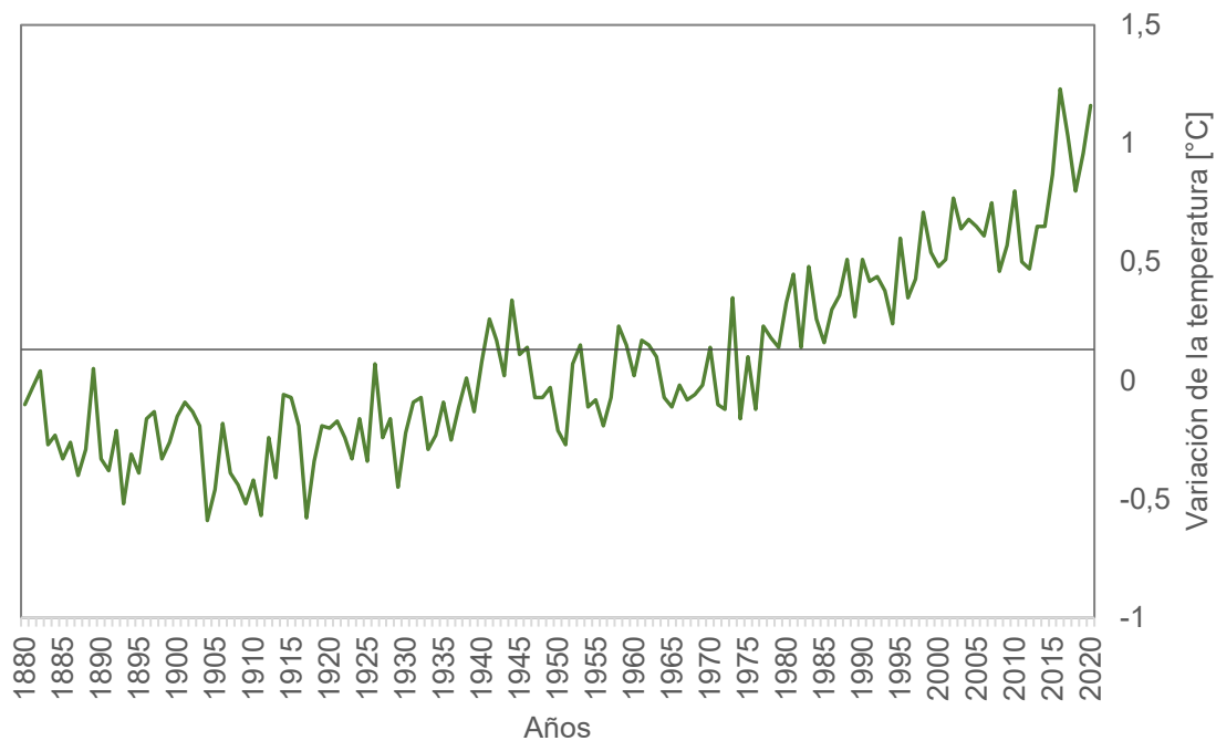
Figura 1. Variación de la temperatura mundial promedio respecto a la era preindustrial. Fuente: Climate.Gov (2022): Climate Change: Global Temperature
