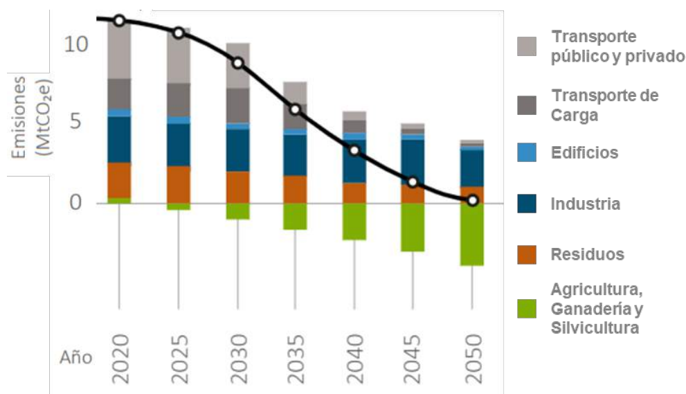
Figura 6. Reducción de emisiones de Costa Rica a 2050. Fuente: Dirección de Cambio Climático, MINAE (2019): Plan Nacional de Descarbonización 2018-2050
