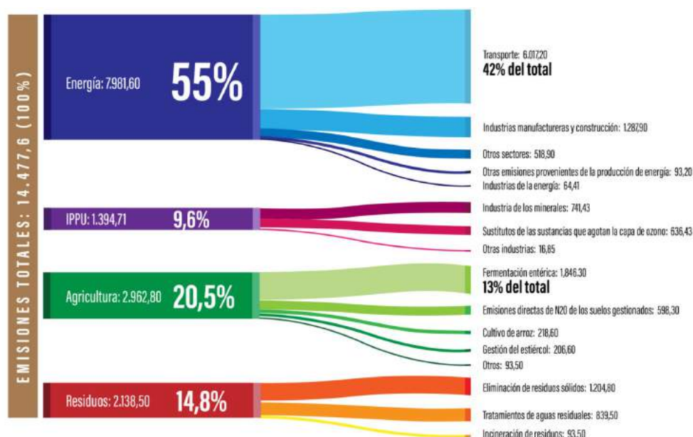
Figura 5. Inventario Nacional de Emisiones de GEI de Costa Rica (Gg de CO 2eq ). Fuente: MINAE (2021): Nuevo Inventario Nacional de Gases de Efecto Invernadero
